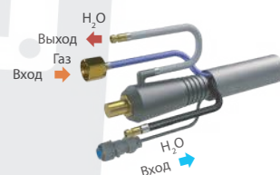
ОКС, М10х1 (вход газ), 6/p (выход H 2 O, вход H 2 O), 7 pin
