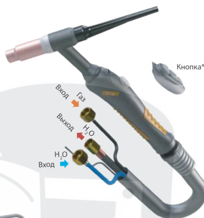
М12х1 (выход H 2 O), 1/4G (вход газ), 3/8G (вход H 2 O)
