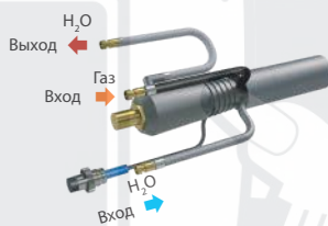
ОКС+6/p (выход H 2 O, вход газ, вход H 2 O), 2 pin
